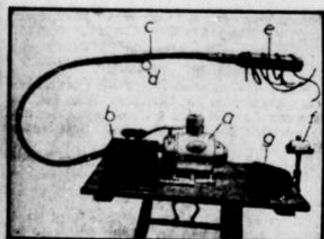
Abb. 1: Elektrische Klopf- und Bürstmaschine. a) Elektromotor mit angebautem Getriebe. b) Regulieranlasser zum Verändern der Drehzahl. c) Biegsame Welle. d) Kettengang mit Momentenhalter zum An- und Abschalten. e) Klopfbürste. f) Spannbügel für das Handstück zum Feststellen des Klopfbereiches. g) Reinigungsbürste.
