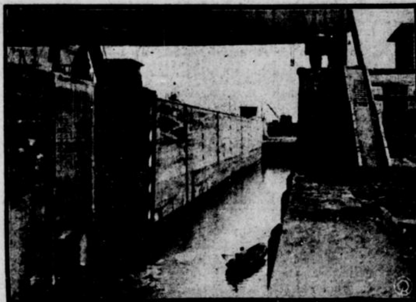
Die großen Schleusen-Anlagen bei Kasselberg ermöglichen eine Verbindung für die Dampfschiffahrt bis nach Mülheim und sind von großer wirtschaftlicher Bedeutung für das Ruhrgebiet. Das Bild zeigt die Schleuse mit dem hydraulisch betriebenen riesigen Eisentor aus der Nähe.
