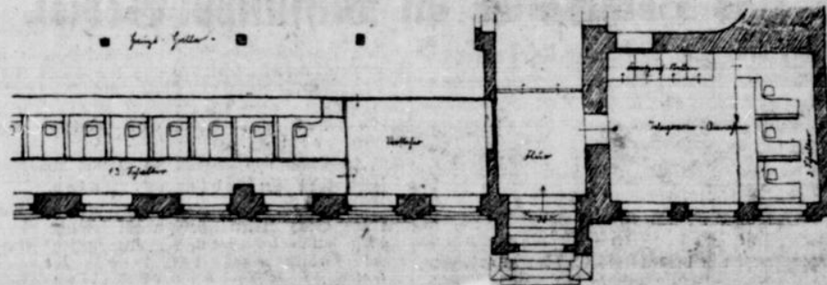
Abb. 2. Grundriß (Teil der Halle und Telegramm-Aufnahme).
