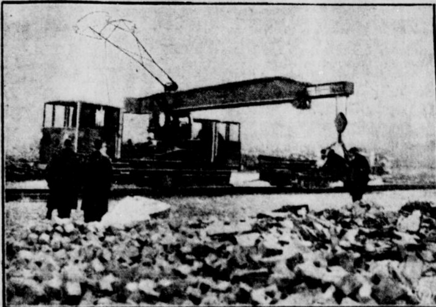
Der Kran zum ersten Male im Gebrauch in den Straßen Kölns.
