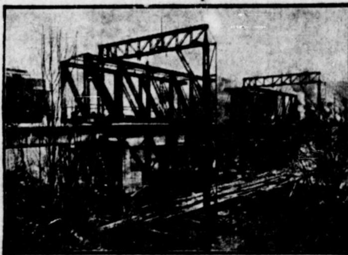
Abb. 2. Der Moment des Abtransportes der alten Heibeker Brücke.
