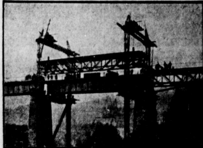
Abb. 3. Umbau der Eisenbahnbrücke bei Krähwinklerbrücke.
