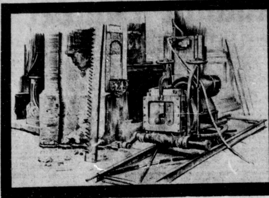
Um Bauwerke vor Zerstörung durch aufsteigende Risse zu schützen, wird das Mauerwerk mit der Mauerfäße durchschnitten und die Schnittfläche mit Bleiplatten isoliert.
