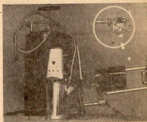
Eine Auswahl aus der großen Kollektion. Das kleinste Lötgerät für den Bastler (im Kreis), ein mittleres und ein großes 50-Liter-Gerät für den Straßenbau.
