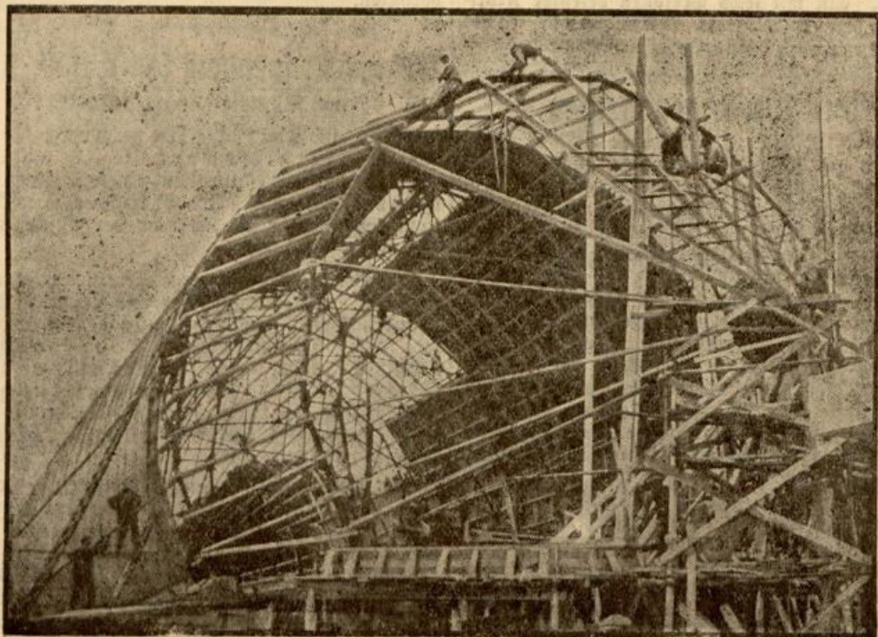
Eine Sternwarte auf dem Pariser Weltausstellungsgelände. Die eigenartige Form dieser auf der Weltausstellung in Paris im Bau befindlichen Sternwarte erinnert an die eines Luftschiffes.
