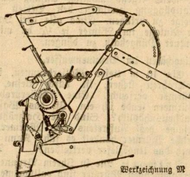
Zeichnung M. Schnitt durch eine Drillmaschine mit Einheitsfärad
