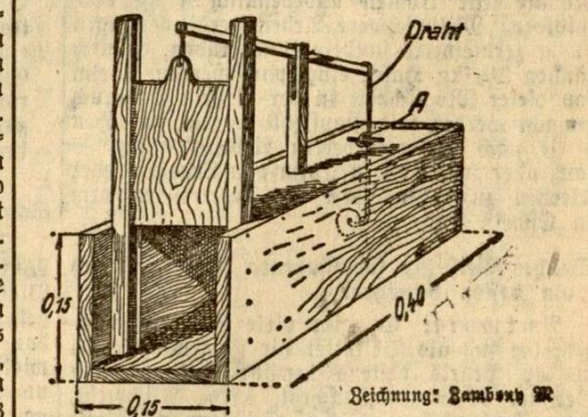
Bezeichnung: Bambus M Rattenfalle
