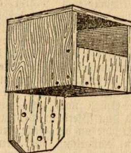
Abbildung 3. Nistkasten für Hausrotschwanz
