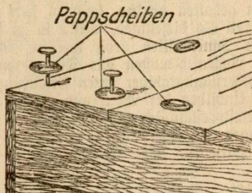
Abbildung 2 Richtiges Anageln von Kisten
