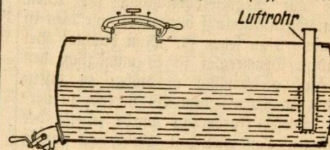
Abbildung 3 Querschnitt durch ein Sauchefäß mit Druckregler
