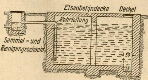
Abbildung 2 Querschnitt durch eine Sauchegrube
