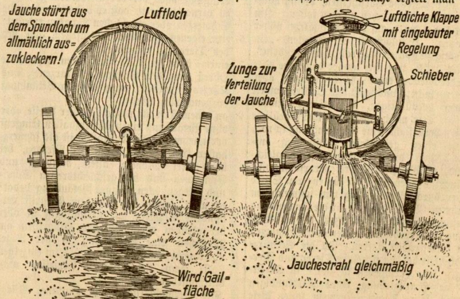
Abbildung 4. Falsche und richtige Saucheverteilung auf dem Acker Links: Falsche Saucheverteilung infolge fehlender Druckregulierung Rechts: Richtige Saucheverteilung infolge Druckregulierung
