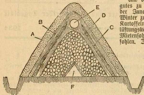
Abbildung 2 Querschnitt durch eine Kartoffelmiete A Verstärkte Erdschicht, B 15-20 cm Kartoffelkraut, C 10 cm Erdschicht, D 15 cm Strohschicht, E Zirkulierung, F Bodenbelag durch Bretterrost
