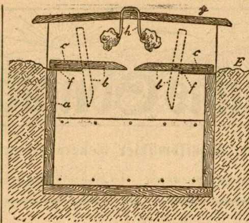
Abbildung 4. Jürnersche Falle für Wühl- und Waldmäuse
