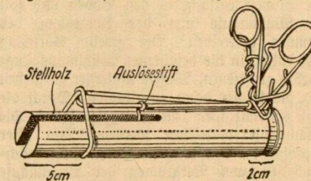
Abbildung 2. Attenkofersche Wühlmausfalle
