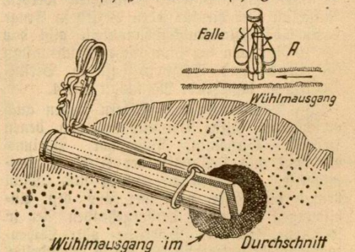
Abbildung 3. Attenkofersche Wühlmausfalle, in einem Wühlmausgang aufgestellt
