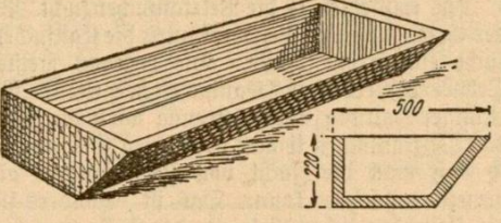
Abbildung 3 Schweinetrog mit einer schrägen und einer geraden Längswand 50 cm außen breit, Längen 50 bis 150 cm
