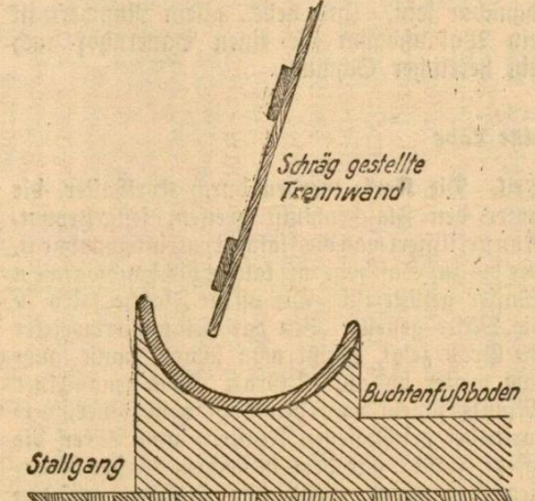
Abbildung 2 Nach innen schräg gestellte Trennwand, um ein Hochklettern der Schweine zu verhindern
