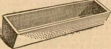
Abbildung 4 Schweinetrog mit vier schrägen Wänden ohne Steg 33 cm außen breit, 19 cm außen hoch, Längen 50 bis 125 cm
