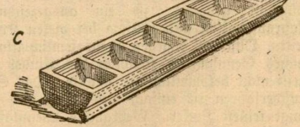
Abbildung 7. Ferkelttröge (Leistentröge) Lichte Weite 15 und 20 cm, Länge 50 bis 125 cm a Ferkeltrog ohne Abteilungen, b Ferkeltrog mit Abteilungen, c Ferkeltrog mit kleinen Abteilungen
