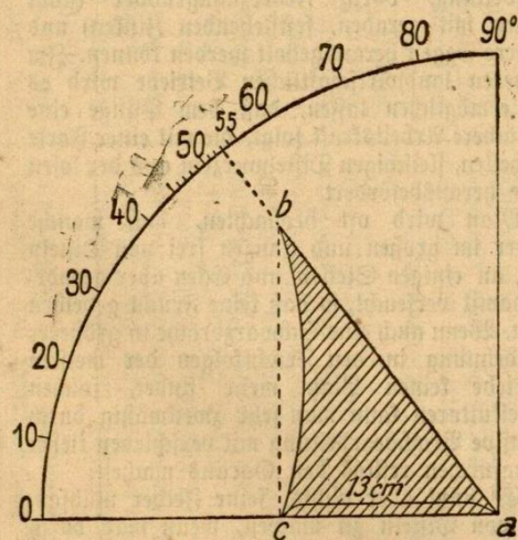
Abbildung 2. Konstruktion des Schattenwerfers für die Sonnenuhr
