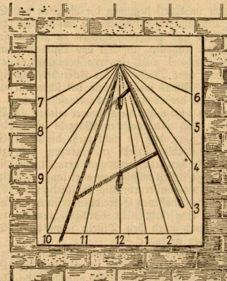
Abbildung 4. Sonnenuhr an der Südwand des Hauses oder der Scheune
