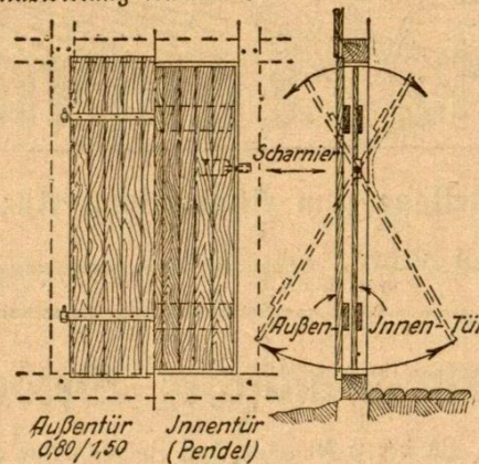
Abbildung 5 Doppeltüren des Weideschuppens Außentüren der Auslaufbuchten.
