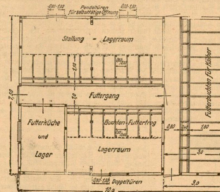
Abbildung 2. Grundriß des Weideschuppens
