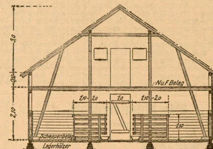
Abbildung 3. Querschnitt des Weideschuppens
