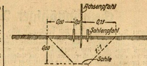
Querschnitt durch den vorschriftsmäßig angelegten Entwässerungsgraben
