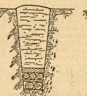
Abb. 5. Stangendrän mit Querholz
