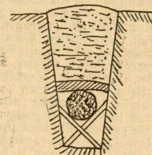
Abb. 3. Fashinendrän auf Holzkreuz
