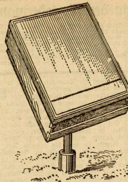
Abbildung 1 Ansicht des Sonnenwachserschmelzers
