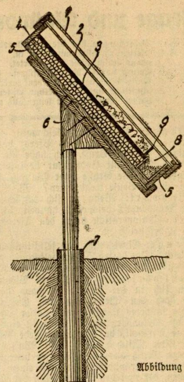
Abbildung 2 Querschnitt des Sonnenwachserschmelzers 1 Glascheibe, 2 Holzleiste, 3 Schieferplatte, 4 Wellpappe, 5 Holzleiste, 6 Blechtrog, 7 Rechen, 8 Röhre eingegraben, 9 Wackstrog, 10 Rechen
