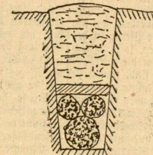
Abb. 2. Drän aus drei Fashinenwürsten
