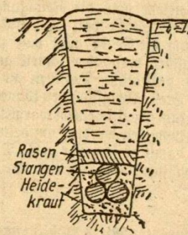
Abb. 4 Stangendrän
