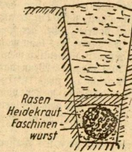
Abb. 1 Fashinendrän
