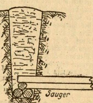
Abb. 6. Verbindung von Sammler und Sauger
