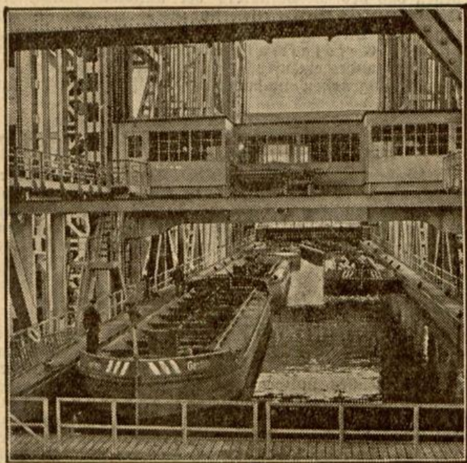
Vor der Eröffnung des größten Schiffshebewerkes der Welt.
