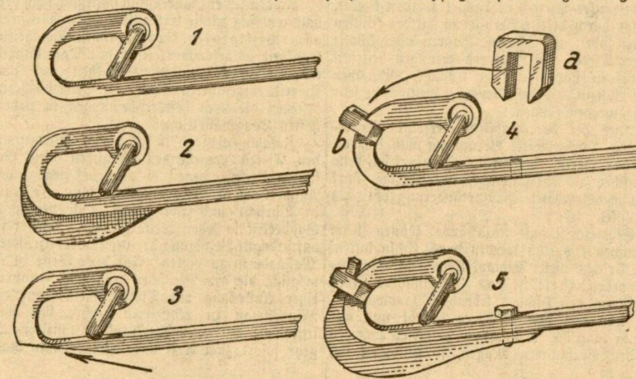
Abb. 1—5. Verschiedene Zughaken an Pflugvorgestellten
