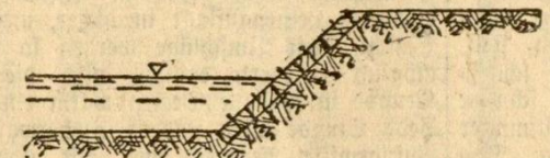
Abbildung 1. Flachrasenbefestigung
