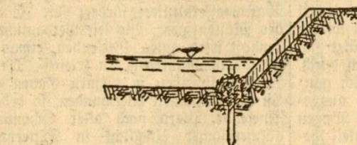
Abbildung 4. Festgenagelte Faschinenwurste
