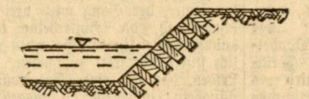
Abbildung 2. Koppfaschenbefestigung
