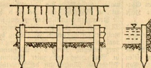
Abbildung 6. Holzschartenwand
