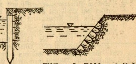
Abbildung 8. Böschungspflaster
