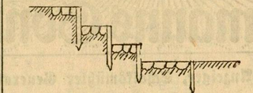
Abbildung 12 Hoher Sohlenabsturz mit Abstößen
