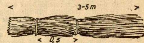
Abbildung 3. Faschinenwurf
