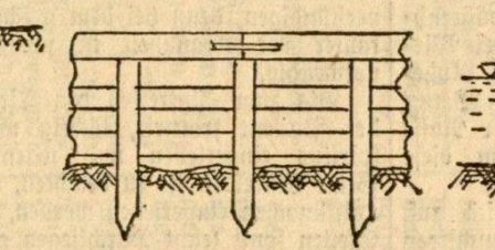
Abbildung 7. Bohlwand
