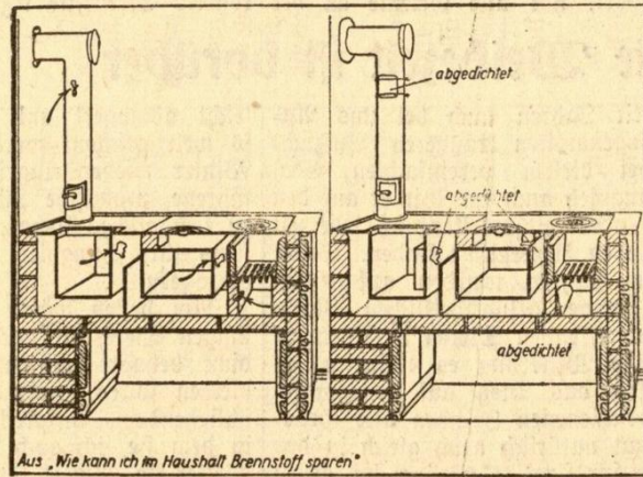
Abbildung 2. Beseitigung von Undichtigkeiten beim Herd
