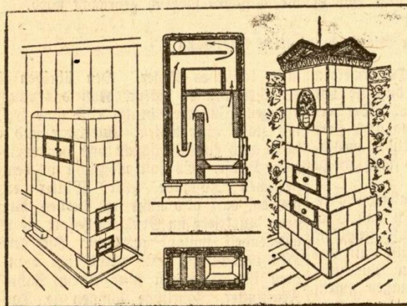
Abbildung 1. Radelofen fest und einfi
