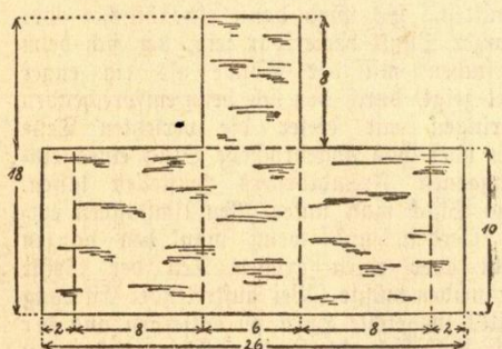
Abbildung 4. So wird das Stück Blech für das Häuschen zugeschnitten
