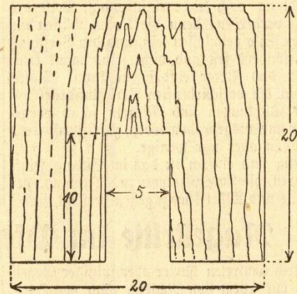
Abbildung 3. Maßzeichnung des Grundbrettchens
