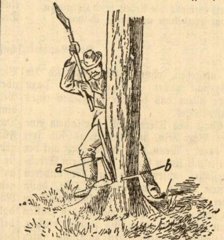
Abbildung 3. Einfagen des Baumes auf der der Fallkerbe gegenüberliegenden Seite
