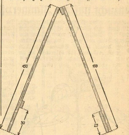
Abbildung 2. Seitenansicht des selbstgebauteen Erd-Durchwurfsiebes
