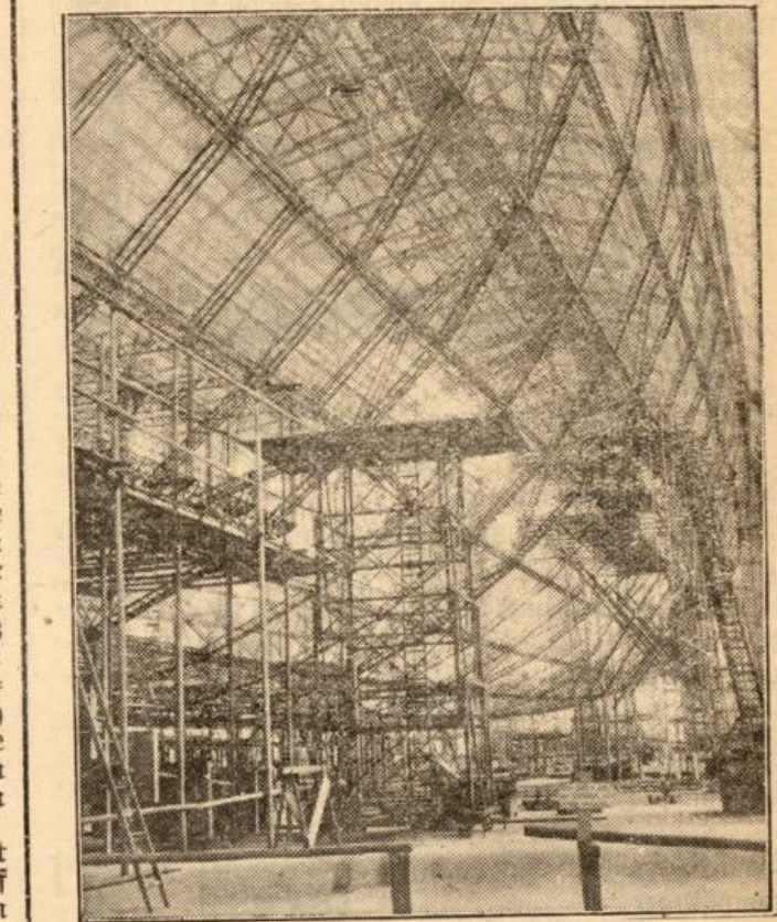
Deutschlands neuer Zeppelin. Unser Bild gibt einen Blick auf das jetzt fertiggestellte Aluminiumgerüst des neuen deutschen Zeppelin-Luftschiffes „Z. 129“ in Friedrichshafen.
