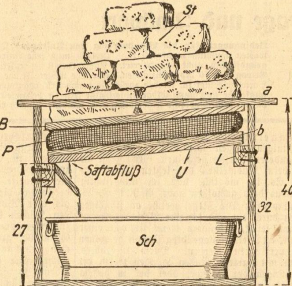
Beerenpresse im Längsschnitt
