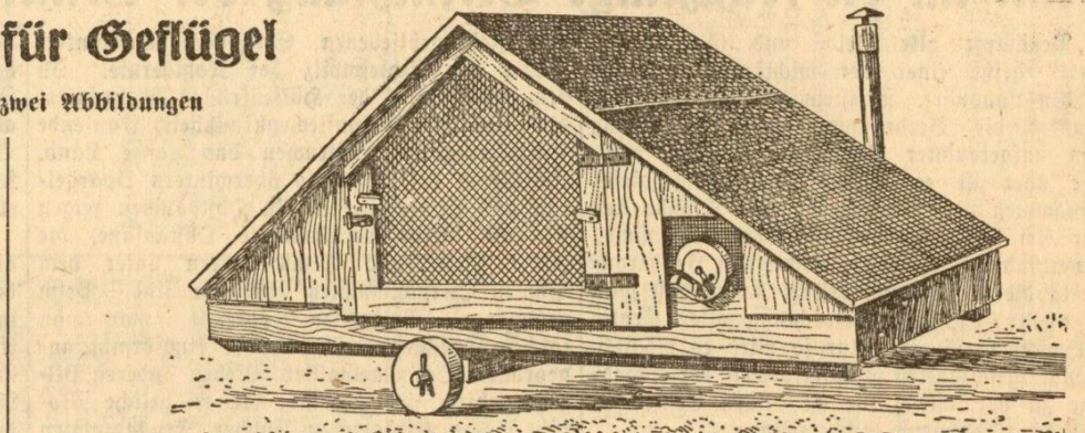
Abbildung 1. Einacher Rollstall für Geflügel, hier als Aufzuchtshaus mit eingebauter Heizung für 100 Küken bestimmt Maße: Länge 2 m, Tiefe 1 m, Firsthöhe 1 m
