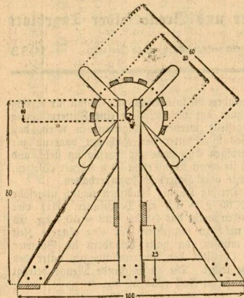
Abbildung 1. Querschnitt der selbstgebauten Gartenschlauchrolle
