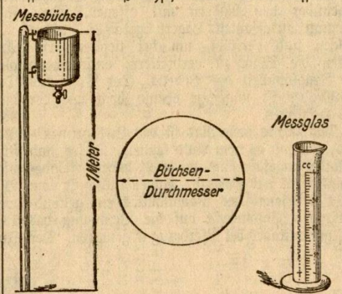
Praktischer Regenmesser
