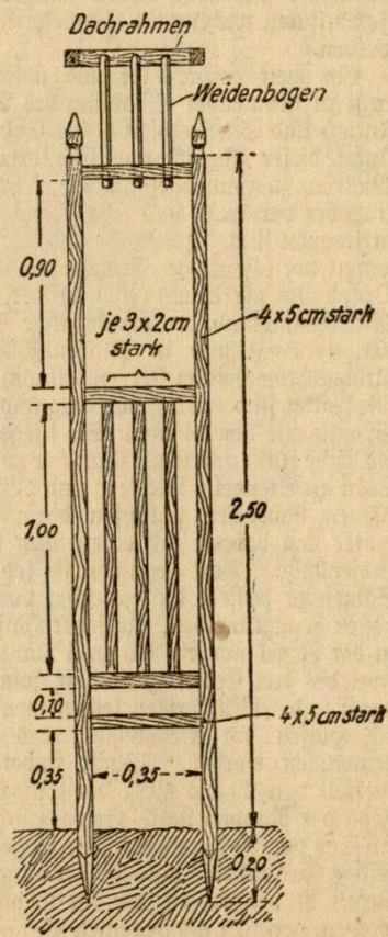
Abbildung 2. Konstruktionszeichnung des Rosenbogens
