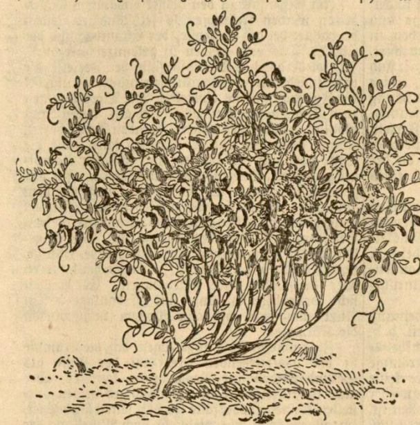
Großkörnige Heller-Linse
