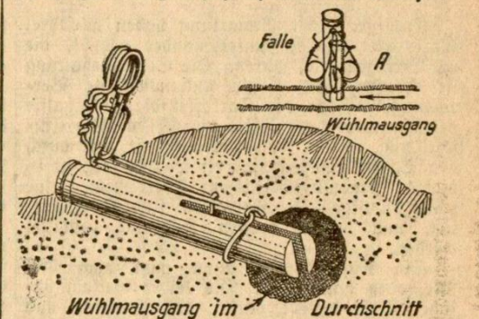
Abbildung 4. Attenkofersche Wühlmausfalle, in einem Wühlmausgang aufgestellt
