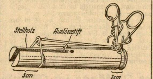
Abbildung 3. Attenkofersche Wühlmausfalle
