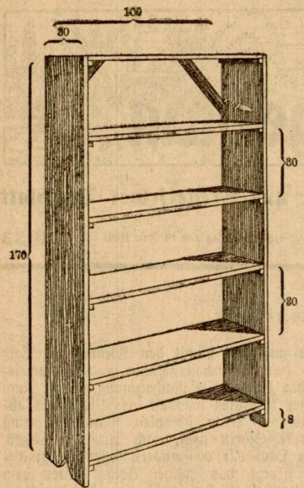
Abbildung 1 Ein Regal für Einmachegläser Die Ziffern sind Maßangaben in Zentimetergröße
