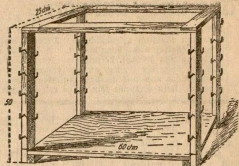
Abbildung 3. Holzernes Gestell zum Auflegen von 18 Drahtnadeln
