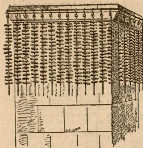
Abbildung 2. Ofensims mit zweckmäßigem Behang von Drahtnadeln, die Obstscheiben zum Trocknen tragen
