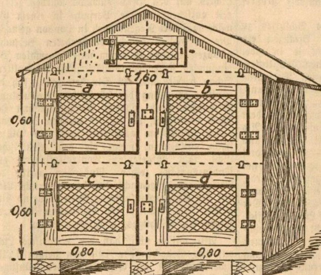
Abbildung 1 Stagenkaninchenstall aus vier gleichgroßen Kästen
