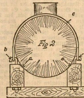
Abbildung 2. Falsche Lagerung wie bei Abbildung 1, aber man hat dem Faß wenigstens eine breitere Auflage gegeben
