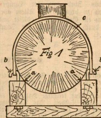
Abbildung 1. Falsche Lagerung. Auflage auf den scharfen Holzkannten, Zugschrauben zu dicht am Faß
