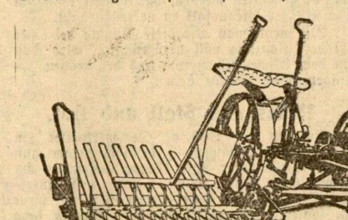
Abbildung 2. Grasmäher mit Handablage.
