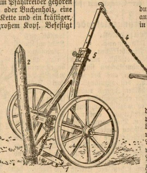
Abbildung 2. Hintergestell eines Aderwagens zum Herausziehen von Zaunpfählen. 1 Querholz des Wagens. 2 Pfahl. 3 Drischel. 4 Zugkette. 5 Wagenarm. 6 Rungenchemel. 7 Eisenkette.
