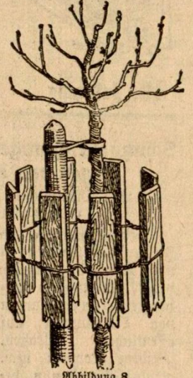
Abbildung 8. Zusammenstellen des Schutzgitters aus Spalierlatten mit Draht.
