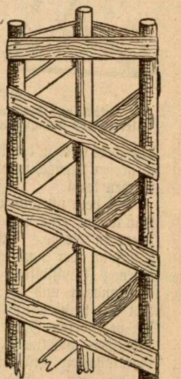
Abbildung 4. Schutzvorrichtung aus Pfählen und Schwarten, die in schräger Anordnung aufgenagelt sind zur Errichtung eines festen Verbandes.
