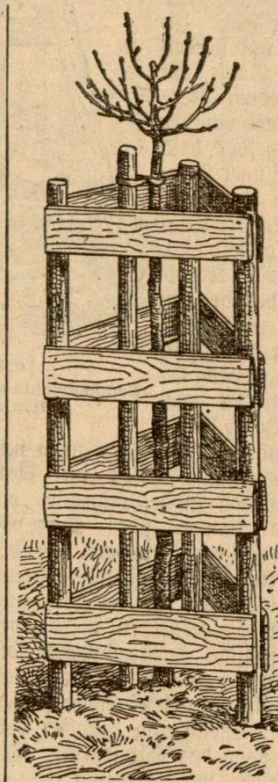
Abbildung 3. Schutzvorrichtung aus Pfählen und Schwarten (dreiteilig).
