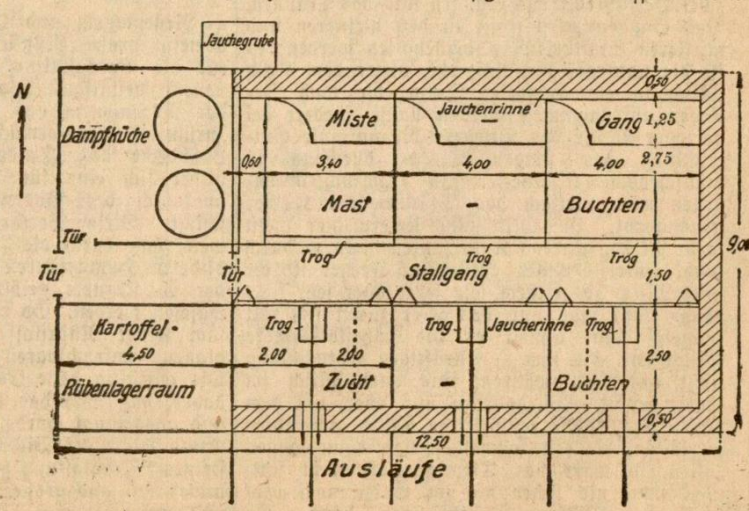
Abbildung 2. Grundriß des Zucht- und Maststalles.
