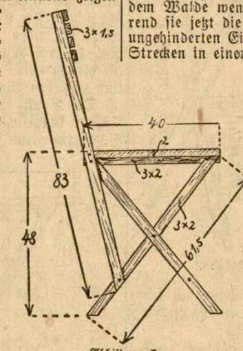
Abbildung 7. Konstruktionszeichnung der Bank und des Stuhles von der Seite.
