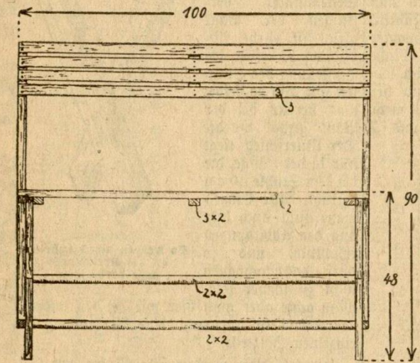
Abbildung 6. Konstruktionszeichnung der Bank von vorn.
