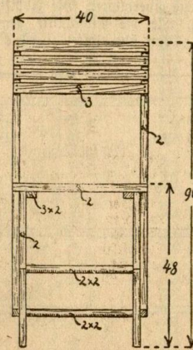
Abbildung 9. Konstruktionszeichnung des Stuhles von vorn.
