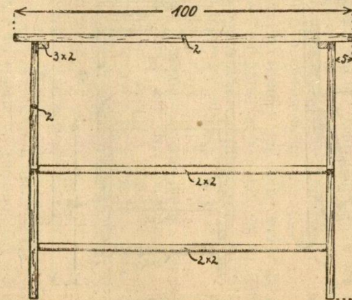
Abbildung 2. Konstruktionszeichnung des Tisches von vorn.
