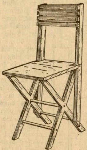
Abbildung 8. Ansicht des Stuhles.
