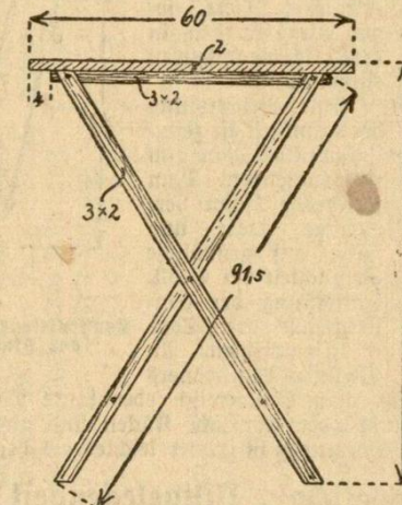
Abbildung 3. Konstruktionszeichnung des Tisches von der Seite.
