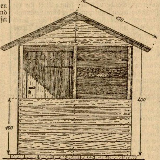
Abbildung 3. Vorderansicht des Gerätehäuschens.
