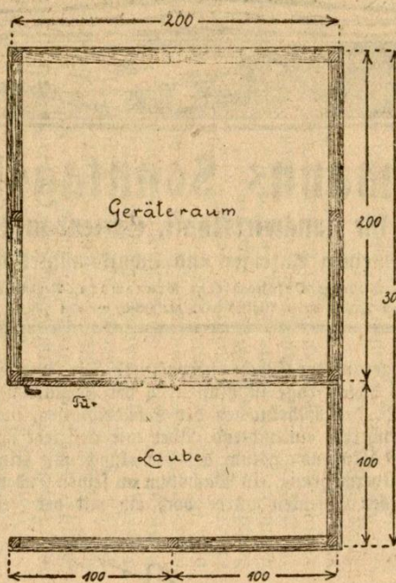
Abbildung 2. Grundriß des Gerätehäuschens.
