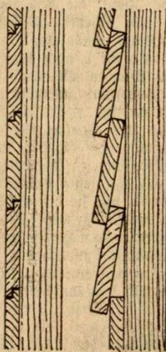
Abbildung 4. Überfalgte oder jaloufiartige geordnete Bretter bilden die äußere Verkleidung.
