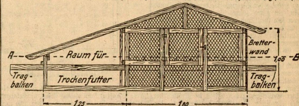
Abbildung 2. Vorderansicht des tragbaren Junggeflügelstalles.
