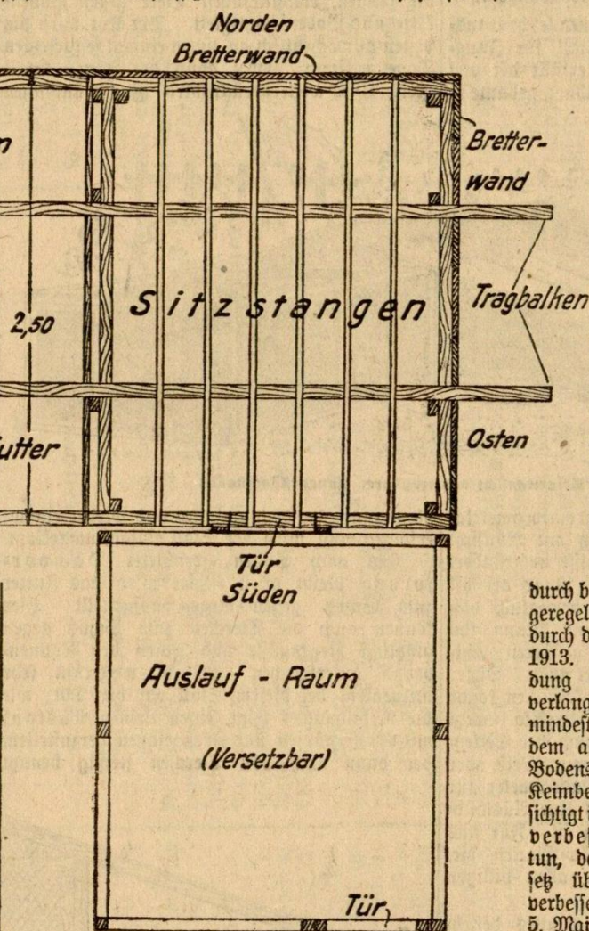
Abbildung 3. Schnitt durch die Linie A-B (Abbildung 2, Vorderansicht) des tragbaren Hühnerklosets.
