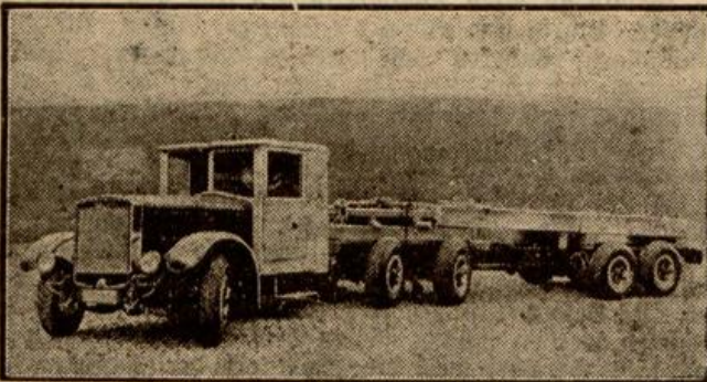
Das größte und schwerste Fahrzeug der Ausstellung ist ein fünfachsiger Krupp-Flettners-Großraum-Lastwagen, dessen „Kettentrigger-Steuerung“ das zweite und dritte Räderpaar automatisch mitsteuert. Das Untergestell, das mit einem 150-PS-Motor ausgerüstet ist, kann eine Nutzlast von 13,7 Tonnen befördern.
