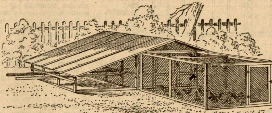
Abbildung 1. Seitenansicht des tragbaren Junggeflügelstalles.
