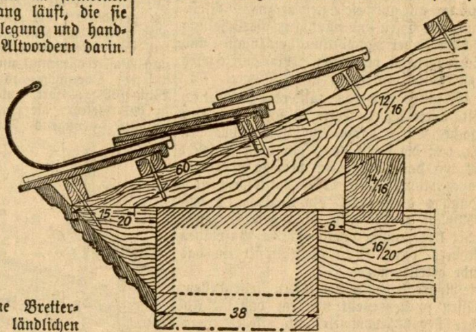
Abbildung 3. Aufgeschraubte Dachrinne.
