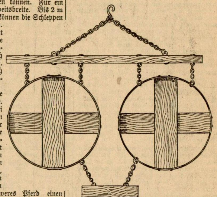
Abbildung 3. Zweiteilige Aderschnelle.
