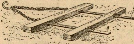
Abbildung 2. Zweiteilige Aderschnelle.
