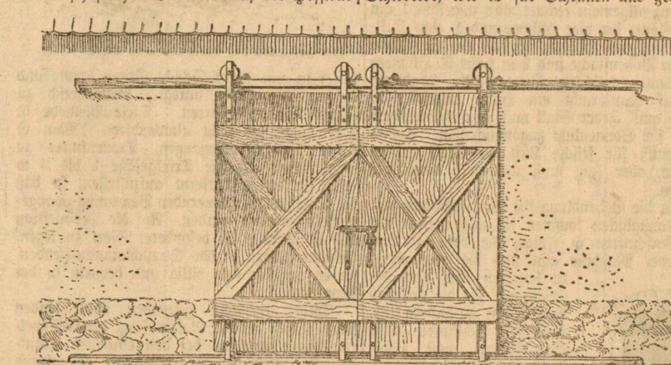
Abbildung 1. Modernes zweiteiliges Schiebtor für Scheunen und größere Ställe.
