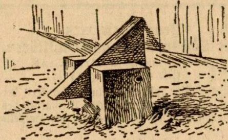
Abbildung 6. Einlader für den Futter- und Wasserkasten der Stalltüren und Scheunentore.
