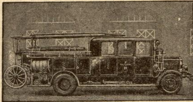
Die neue Konstruktion einer Feuerwehrspritze zeigt einen verdeckten Raum für die Bedienungsmannschaft.
