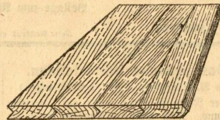
Abbildung 1. Keilspundung.
